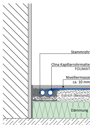
Fußbodenschnitt Kapillarrohrmatte auf Estrich
